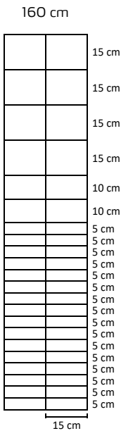
Art.Nr.: 2316002 100 Meter 160cm/23/15 - LIGHT
