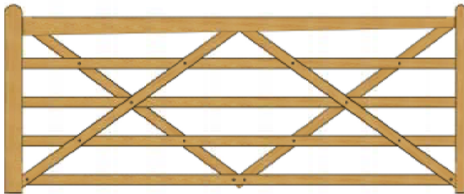
B: 300 cm H: 114 cm
